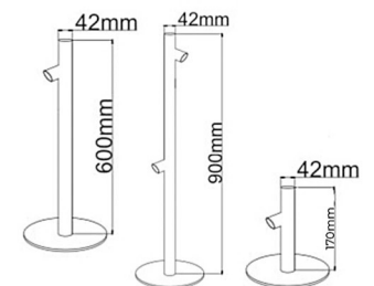
ANKUR SKEZIO BOLLARD 3W/2X3W
